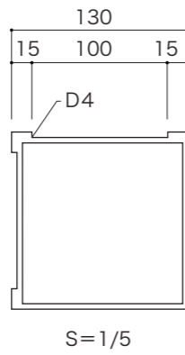
B-B' 断面図
